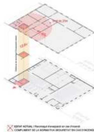
ESQUEMA DEL COMPLIMENT DE LA NORMATIVA D'INCENDIS
